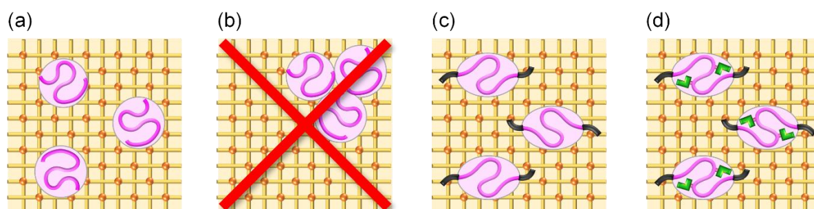
図 2. エポキシ樹脂中でのゴム成分の分散のイメージ. (a) ゴム成分の理想的な均一分散. (b) ゴム成分の凝集. (c) SIS の分散. (d) 水素結合性 SIS の分散. 黄色の線とオレンジのドットは硬化したエポキシ樹脂, ピンクの曲線はゴム成分, 黒色の線はエポキシ樹脂に可溶な高分子成分, 緑色の L 字は水素結合性官能基を表す.
